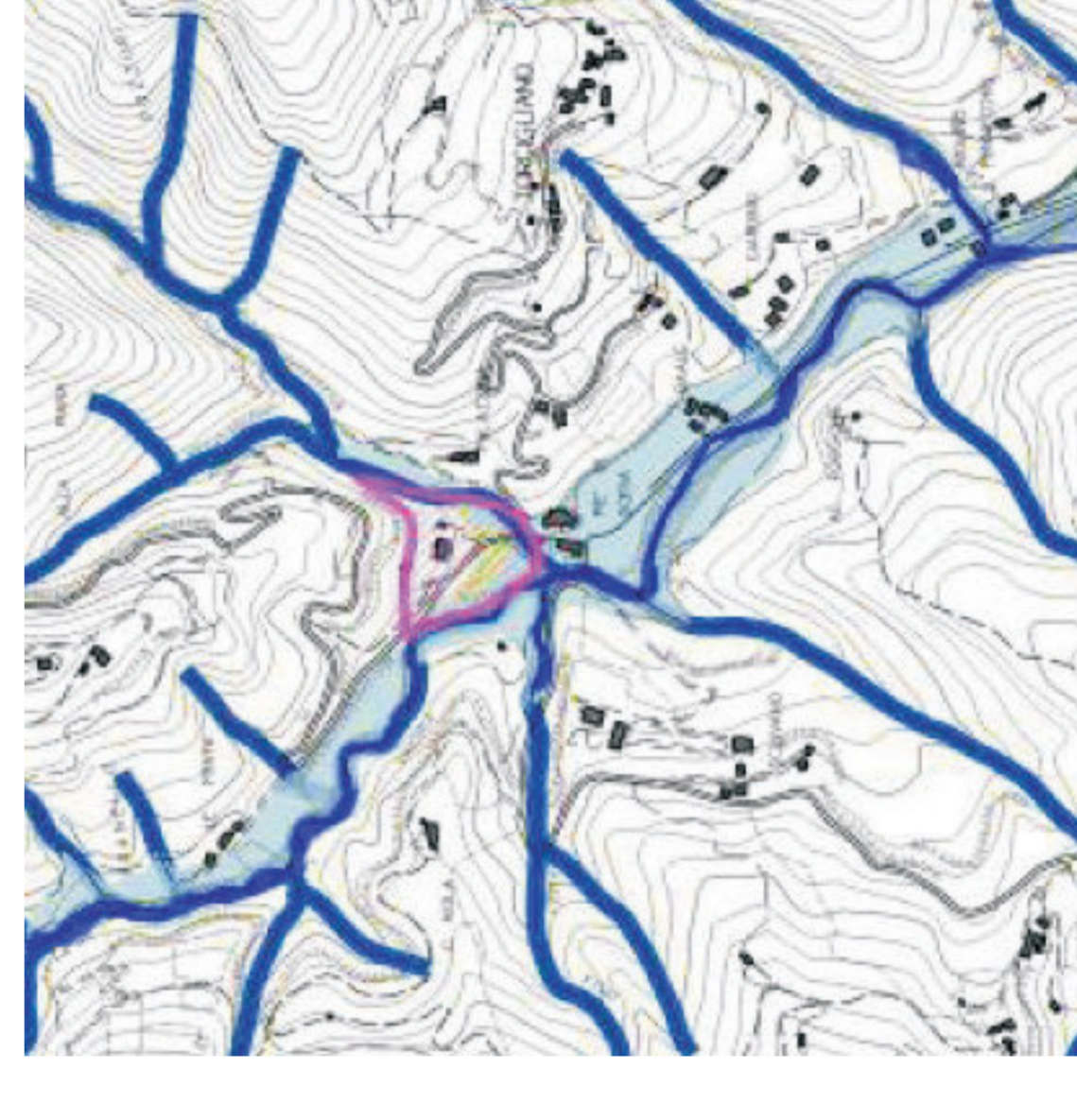
10 Pericolosità idraulica P.S. intercomunale I.3 Pericolosità elevata Scala -
